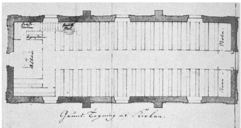
Grundtegning
